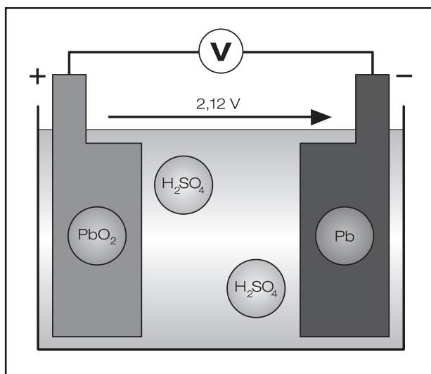
Nabitý článek baterie
